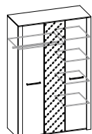
вэд. 3 1492 × 627 × 2216
