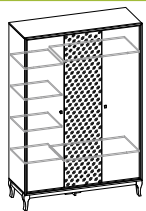
изд. 354 1548 × 596 × 2200
